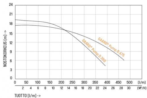
UPPOPUMPPUJEN TUOTTOTAULUKOT N=2860 R/MIN
